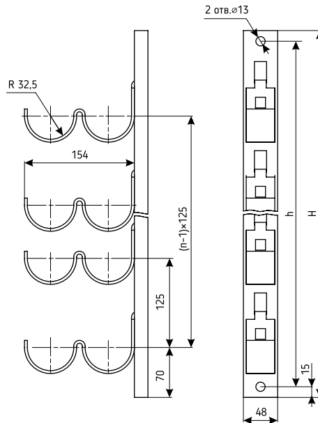
РИС. 1. Кронштейн двухрожковый прямолинейный
